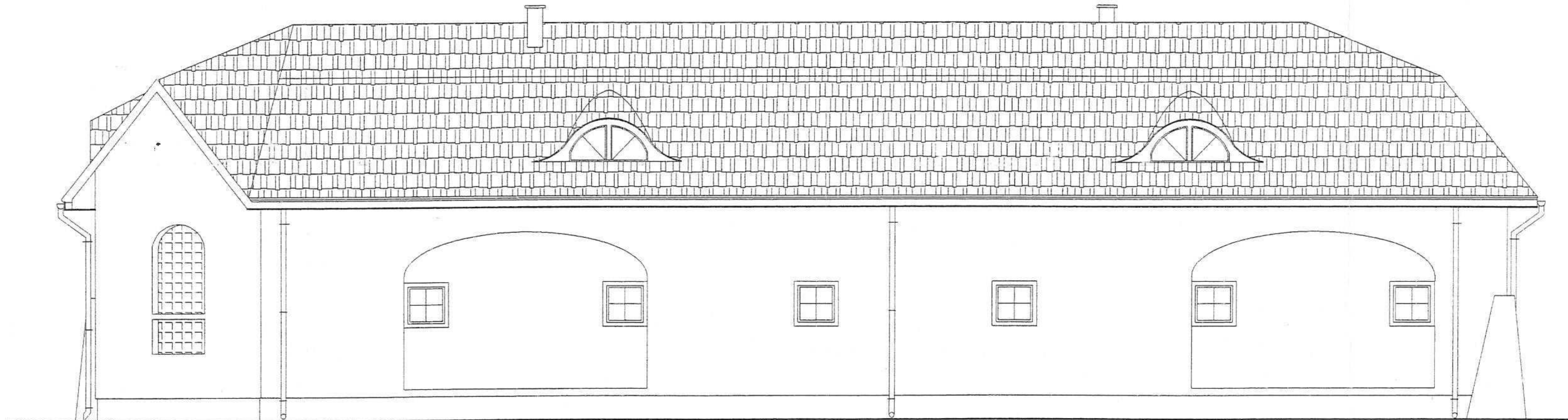
ELEWACJA WSCHODNIA skala 1:100
