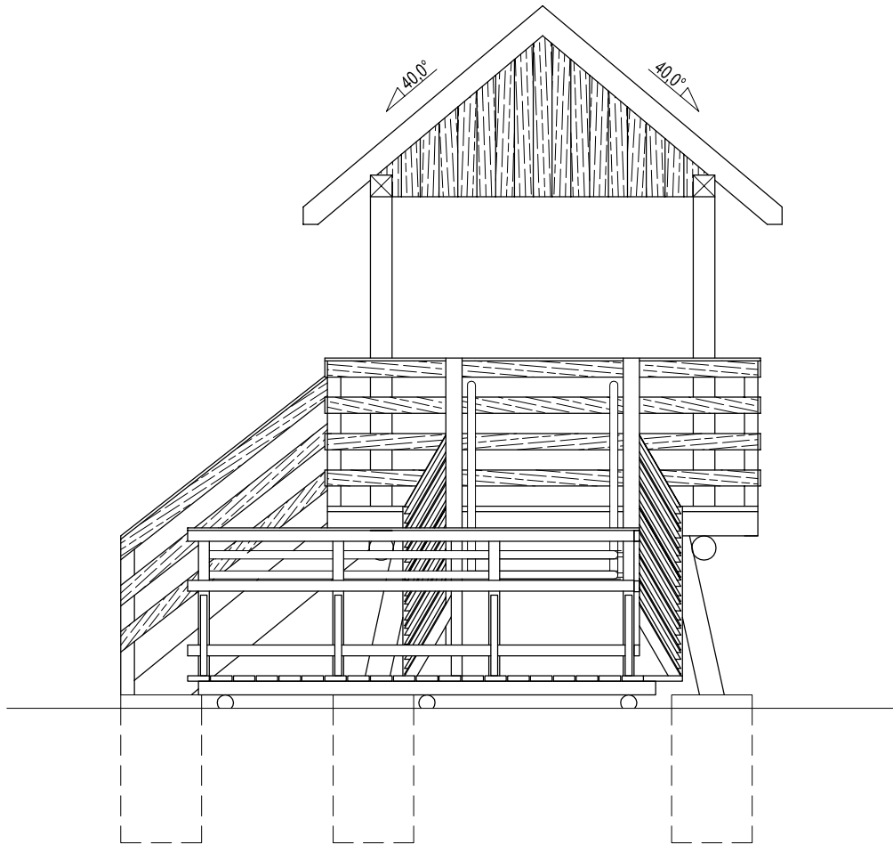
ELEWACJA BOCZNA PRAWA
