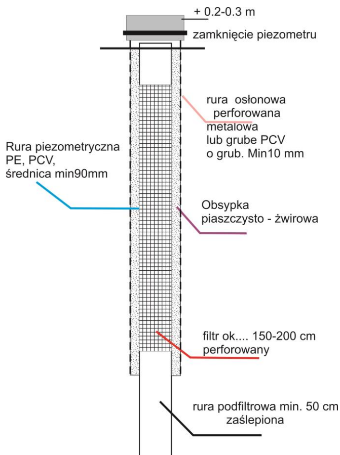
Rycina 2. Schemat wykonania piezometru do pomiarów wód podziemnych.
