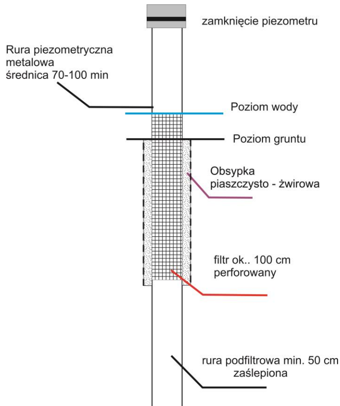
Rycina 1. Schemat wykonania piezometru do pomiarów w ciekach i jeziorach.
